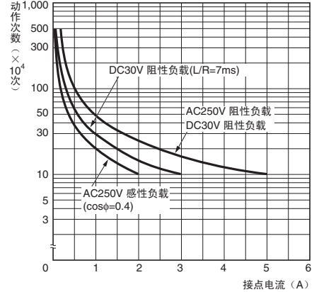
G2R-1Z4、G2R-1AZ4
