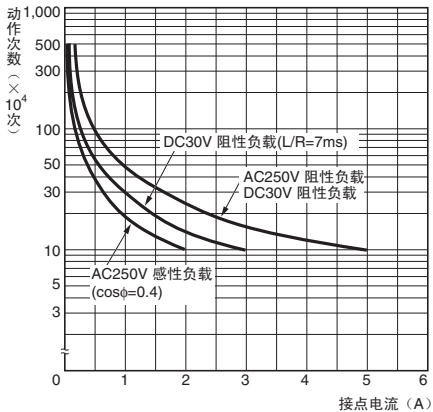
G2R-1-H、G2R-1A-H、G2R-2、G2R-2A
