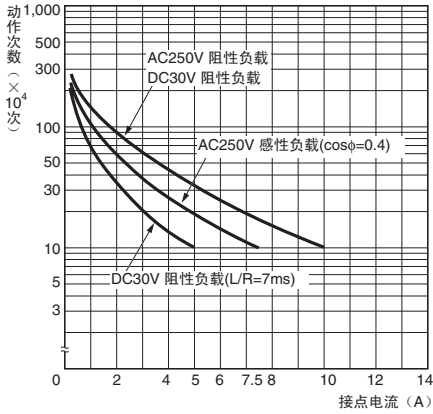
G2R-1-H、G2R-1A-H、G2R-2、G2R-2A
