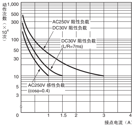
G2R-2-H、G2R-2A-H
