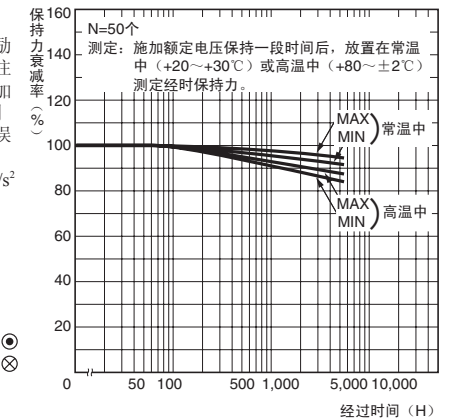
G2RK-1
