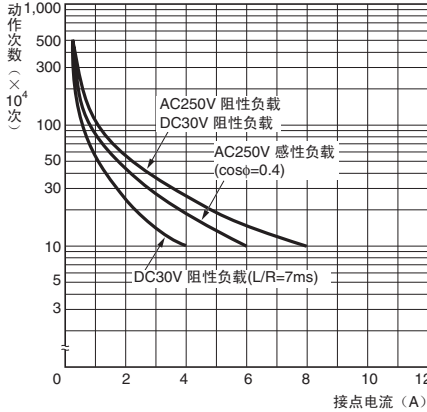
G2R-14、G2R-1A4
