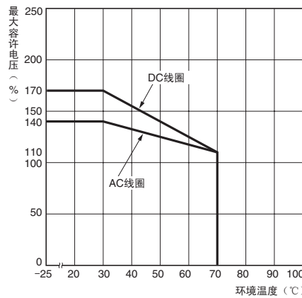
G2R-1 N=5个
