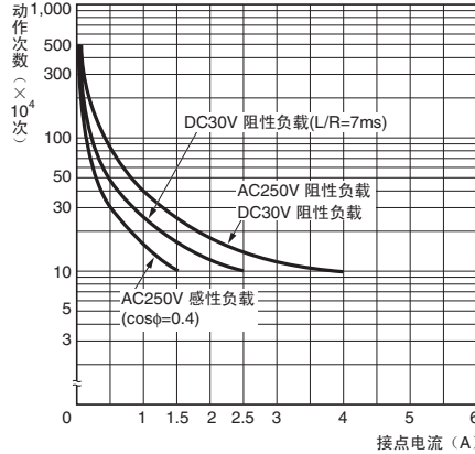
G2R-24、G2R-2A4
