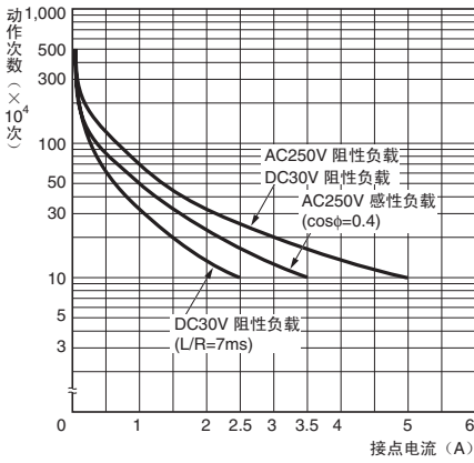
G2RK-1A、G2RK-1
